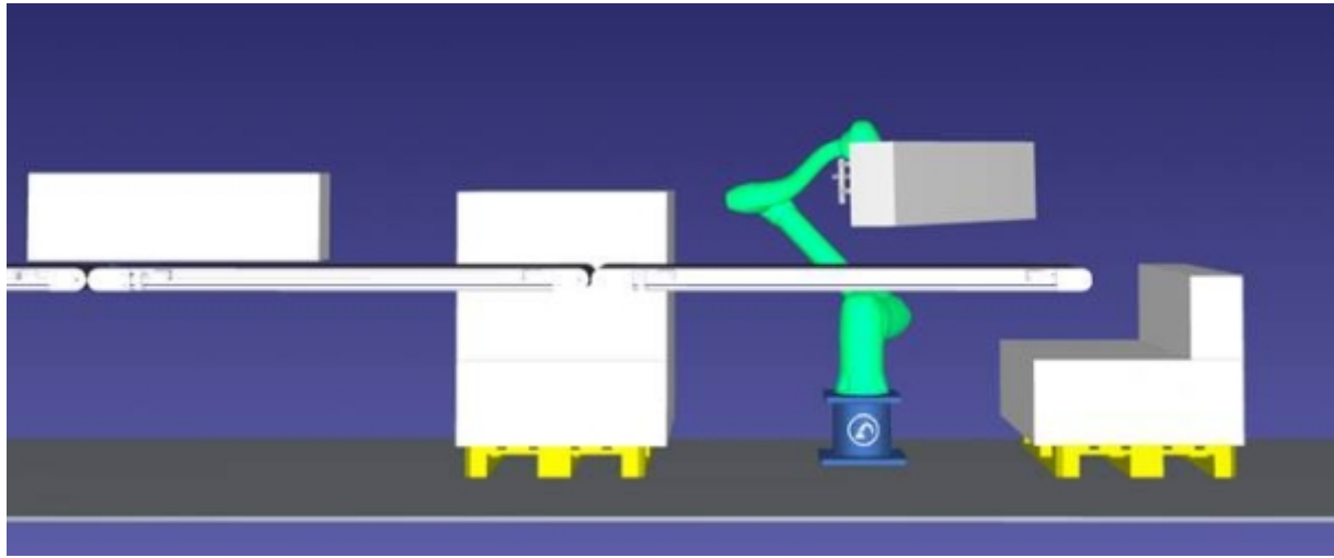
Figure 2 : simulation de palettisation simple avec RoboDK - temps de programmation : 1 heure
