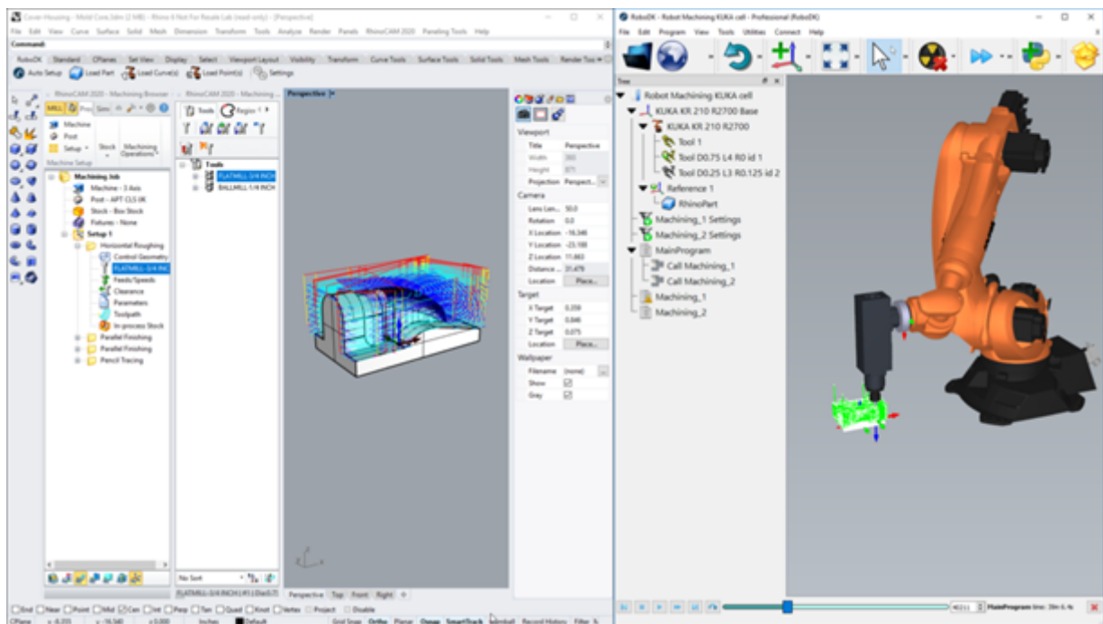
Figure 5 : Application de fraisage RoboDK avec plug-in Rhino CAM
