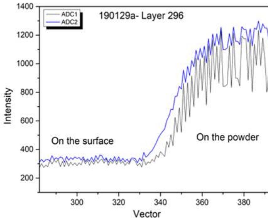
Illustration 2 : exemple d'un fichier de sortie d'un système MPM pour la SLM, qui montre la sensibilité du signal aux conditions de production (scan sur surface fondue vs. scan sur poudre)
