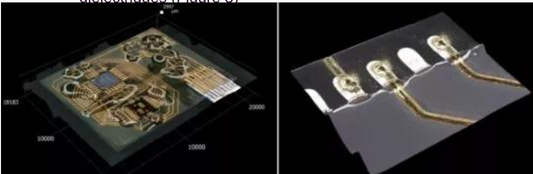
Figure 3 - Vue (microscope optique 3D) du circuit final, y compris zones de croisement (gauche) et détail de la circuiterie micro- imprimée dans une zone de transition substrat-composant
