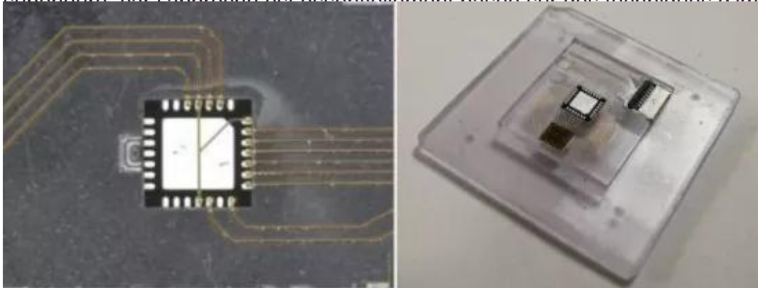
Figure 1 - Intégration et interconnexion de composants électroniques sans PCB dans des substrats imprimés 3D (3D-PID)
