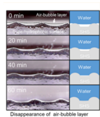
Evolution d'une surface superhydrophobe en immersion.
