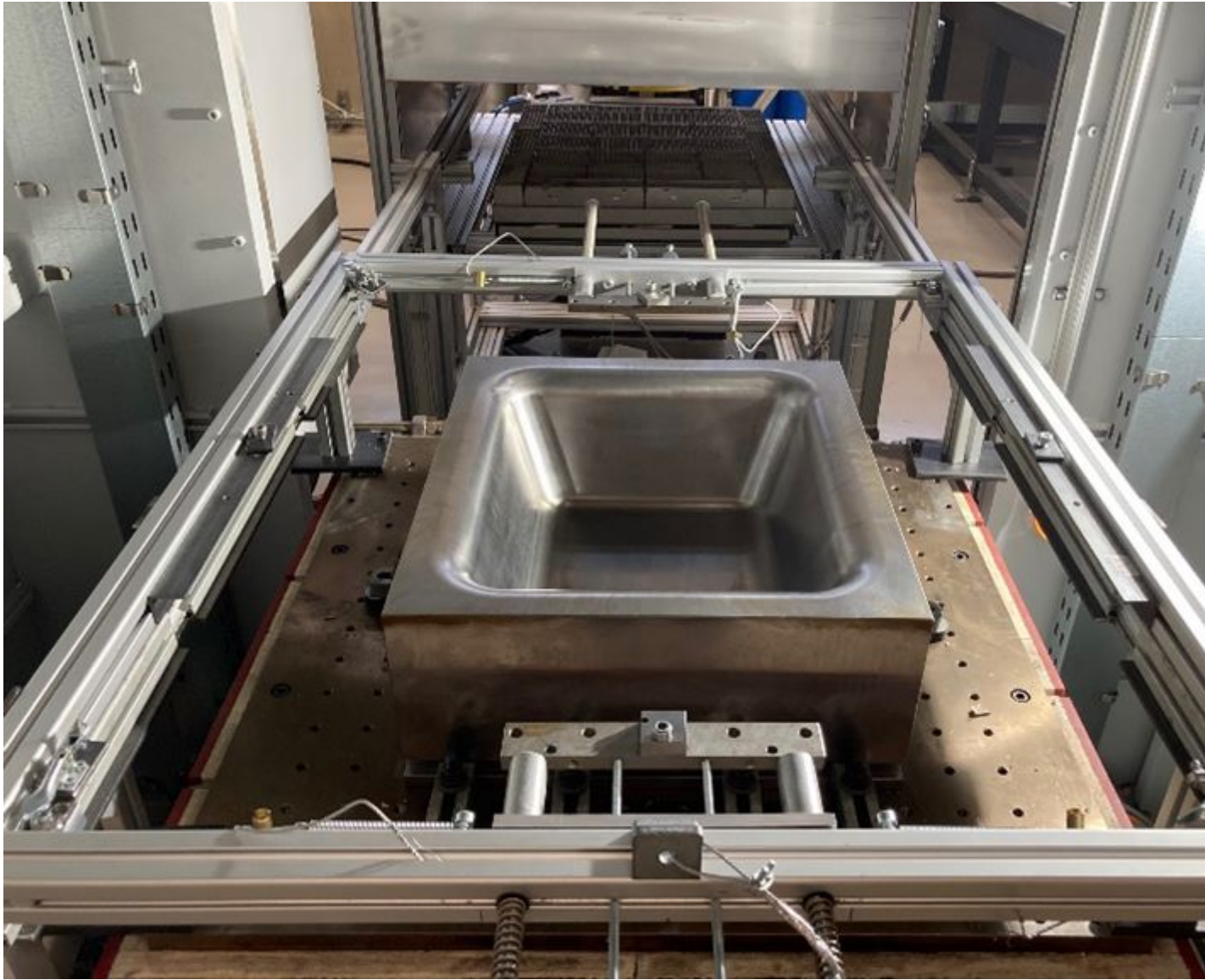
Figure 7 : configuration de la presse visant à presser une cuvette à partir d'une plaque consolidée
