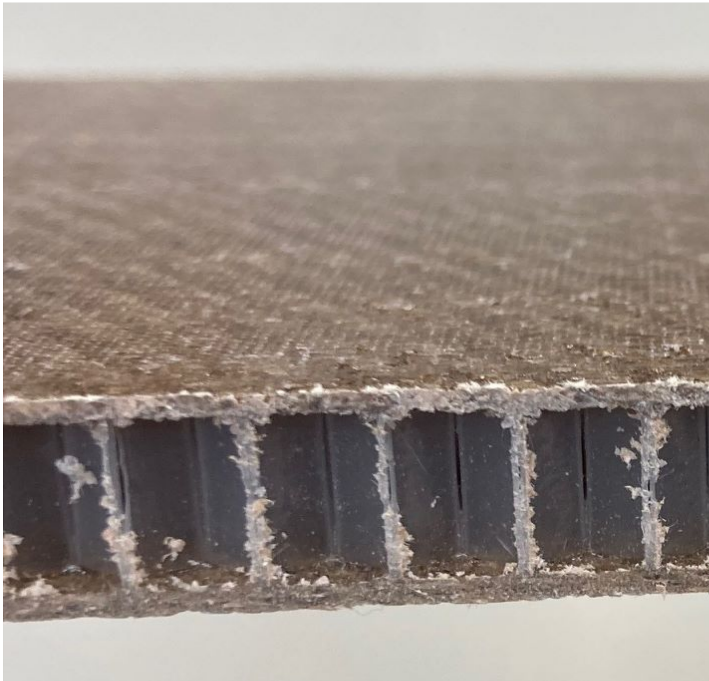
Figure 1 : exemple de structure en sandwich PLA-lin
