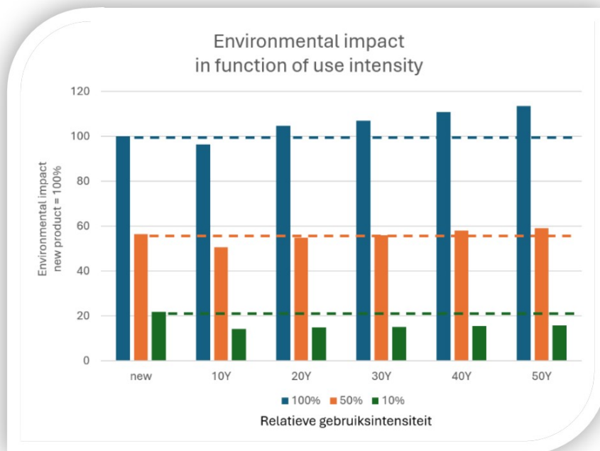
Figure 3 : influence de l'intensité d'utilisation sur les avantages environnementaux ReX d'un produit plus ancien
