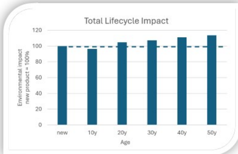
Figure 2 : impact total sur le cycle de vie d'un produit remanufacturé par rapport à un produit neuf
