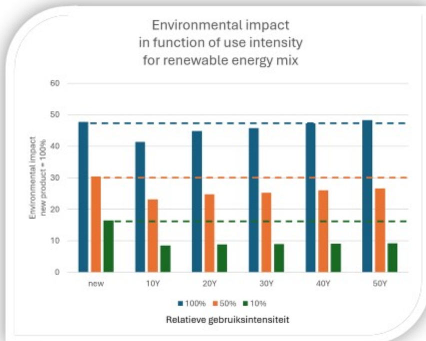
Figure 4 : impact environnemental relatif du remanufacturing dans une région où la part des énergies renouvelables est élevée (Norvège)
