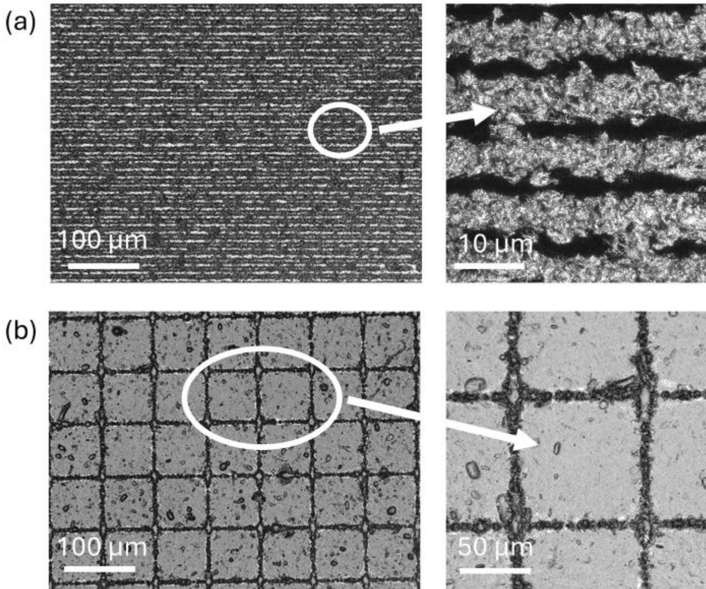
Figure 2. Revêtements en nanocellulose texturés au laser pour créer (a) des motifs unidimensionnels, (b) des motifs bidimensionnels. Limitée par le diamètre du faisceau laser, la taille minimale des motifs s'élève à 15 µm.
