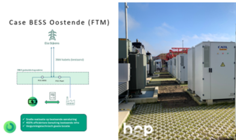
Figure 2: cas BESS à Ostende
