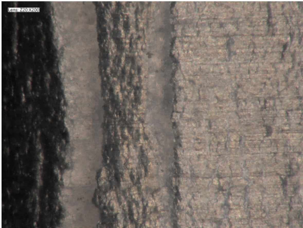
Figure 6 : les images au microscope des échantillons de revêtement A non vieilli et vieilli montrent que les membranes de revêtement sur le substrat se fissurent à T0.
