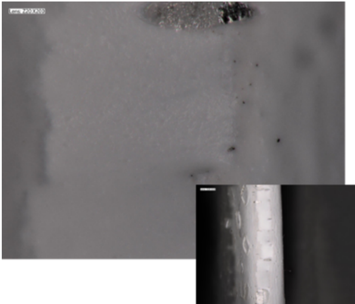
Figure 7 : les images au microscope des échantillons de revêtement D non vieilli et vieilli montrent que le revêtement se déchire à T0.
