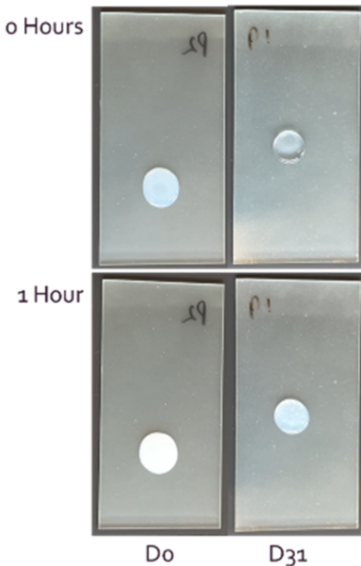
Figure 10 : photographies des échantillons de revêtement P non vieilli et vieilli à différents intervalles pendant l'essai de résistance chimique.
