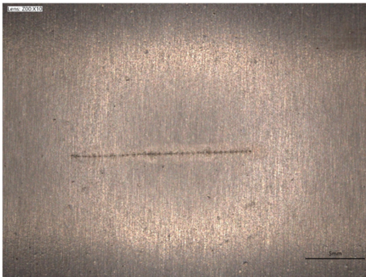
Figure 9 : images au microscope de la rayure sur les échantillons de revêtement P non vieilli et vieilli.
