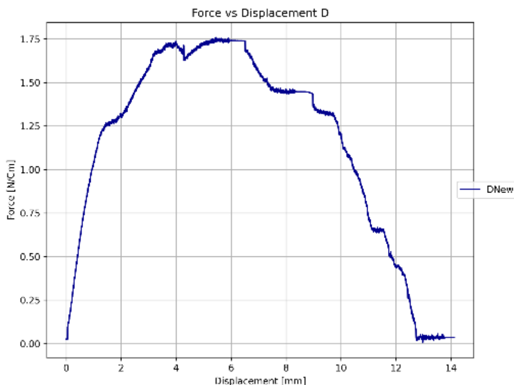
Figure 4 : courbe force-déplacement issue de l'essai de pelage réalisé sur le revêtement D.
