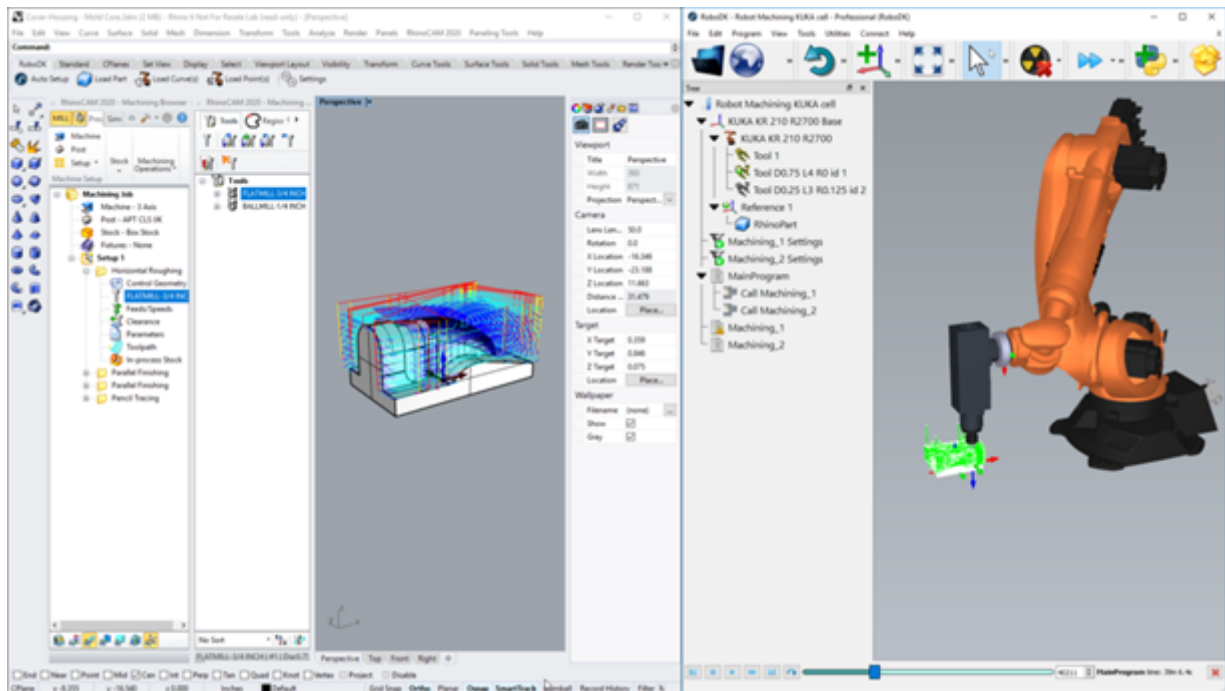
Afbeelding 5: een freestoeppassing van RoboDK met Rhino CAM plug-in
