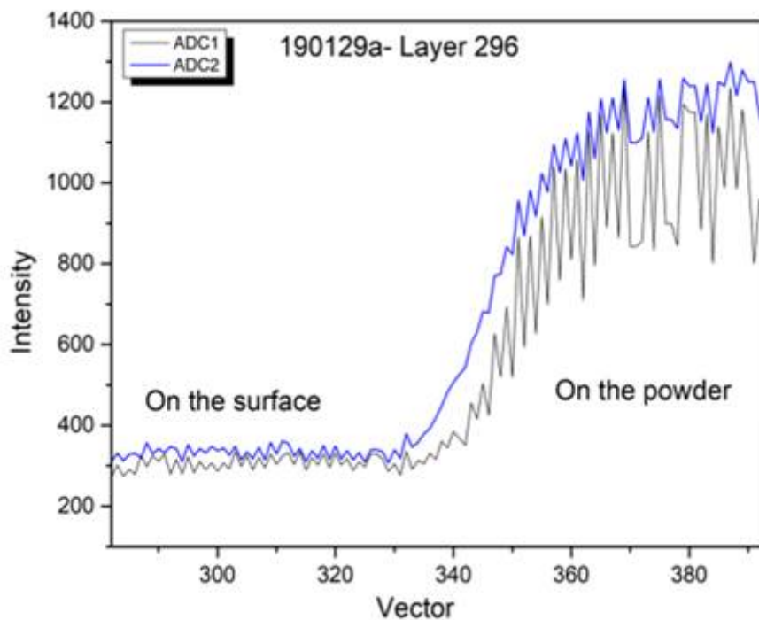
Figuur 2: Voorbeeld van een outputbestand van MPM-systeem voor SLM, dat de gevoeligheid van het signaal voor productieomstandigheden toont (scan op gesmolten oppervlak vs. scan op poeder)
