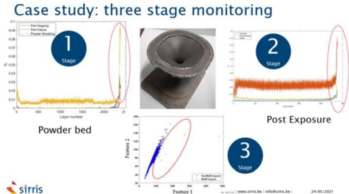
Figuur 3: Geautomatiseerde anomaliedetectie door gebruik te maken van machine learning, toegepast in een casestudy op een stuk dat als benchmark diende
