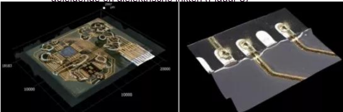
Figuur 3 - Aanzicht (optische 3D-microscoop) van het uiteindelijke circuit, inclusief overgangsgebieden (links) en detail van de microgeprinte schakelingen in een overgangsgebied van een substraatcomponent
