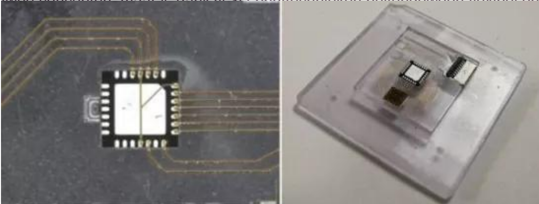
Figuur 1 - PCB-loze integratie en onderlinge verbinding van elektronische componenten in 3D-geprinte substraten (3D-PID)
