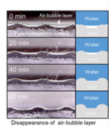
Tijdelijk karakter van ondergedompeld superhydrofoob oppervlak.
