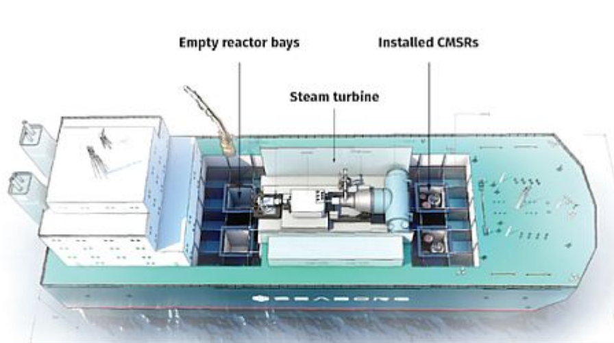
©Seaborg Afbeelding 3: CMSR Power Barge concept
