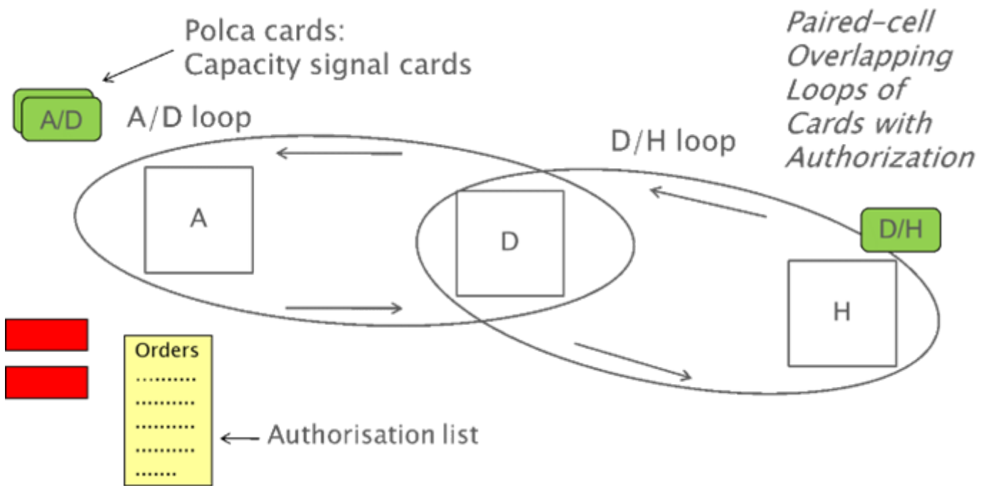
Figuur 1 Twee overlappende POLCA-lussen met POLCA-kaarten
