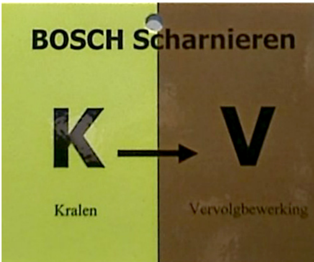
Figuur 2 POLCA-kaarten van Bosch Scharnieren
