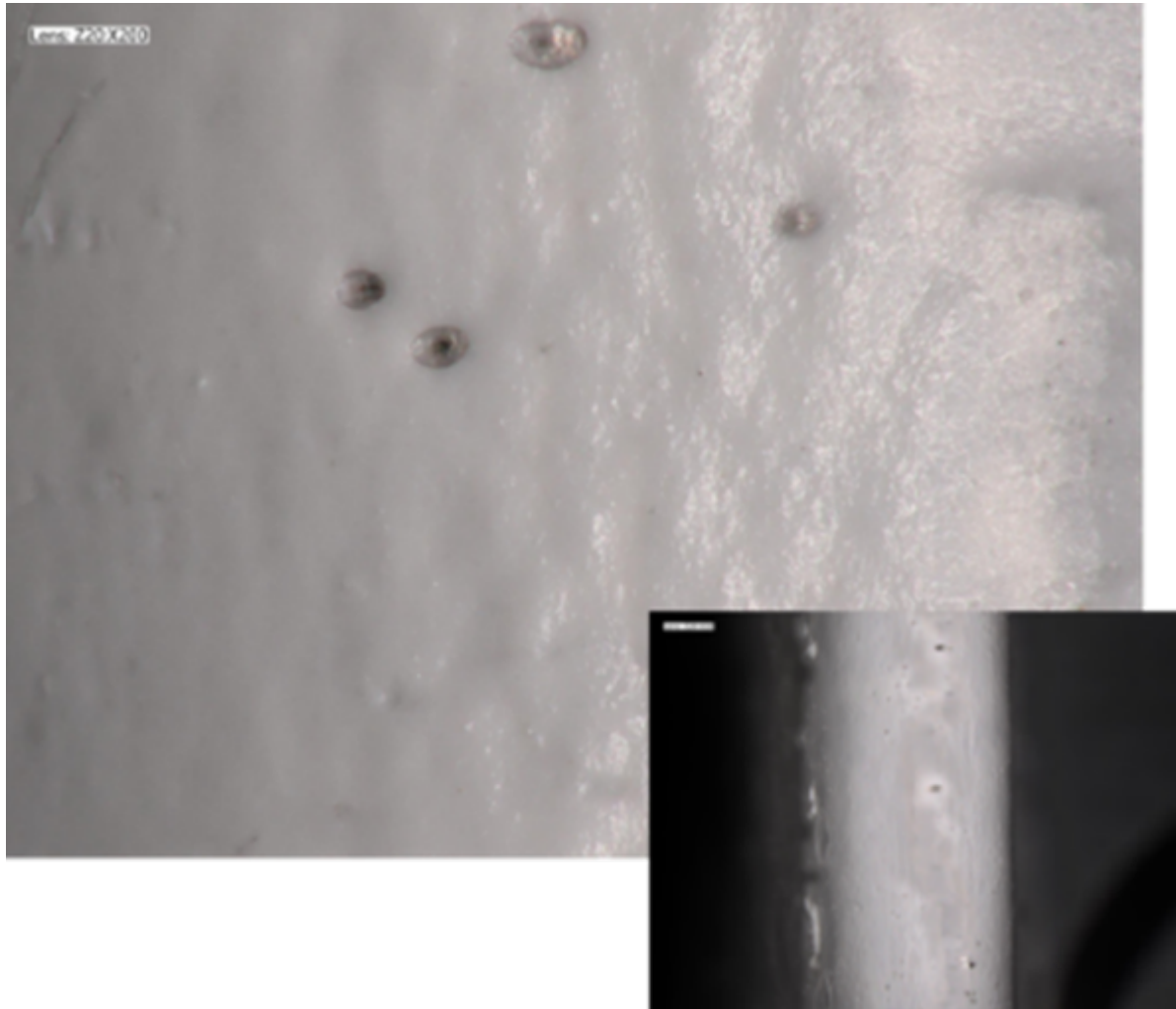
Figuur 8 microscopische beelden van de niet-verouderde en verouderde monsters van Coating D laten zien dat de coating intact blijft bij T1.
