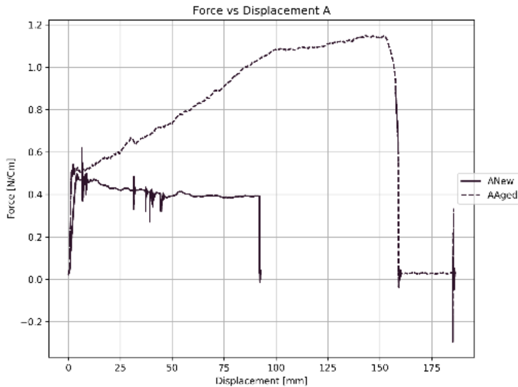
Figuur 2: krachtverplaatsingscurven van de afpeltests uitgevoerd op Coating A.
