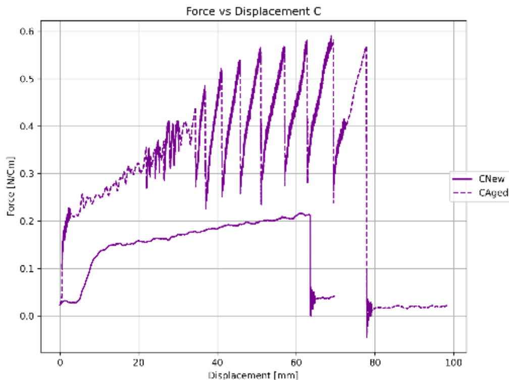
Figuur 3: krachtverplaatsingscurven van de afpeltests uitgevoerd op Coating C.
