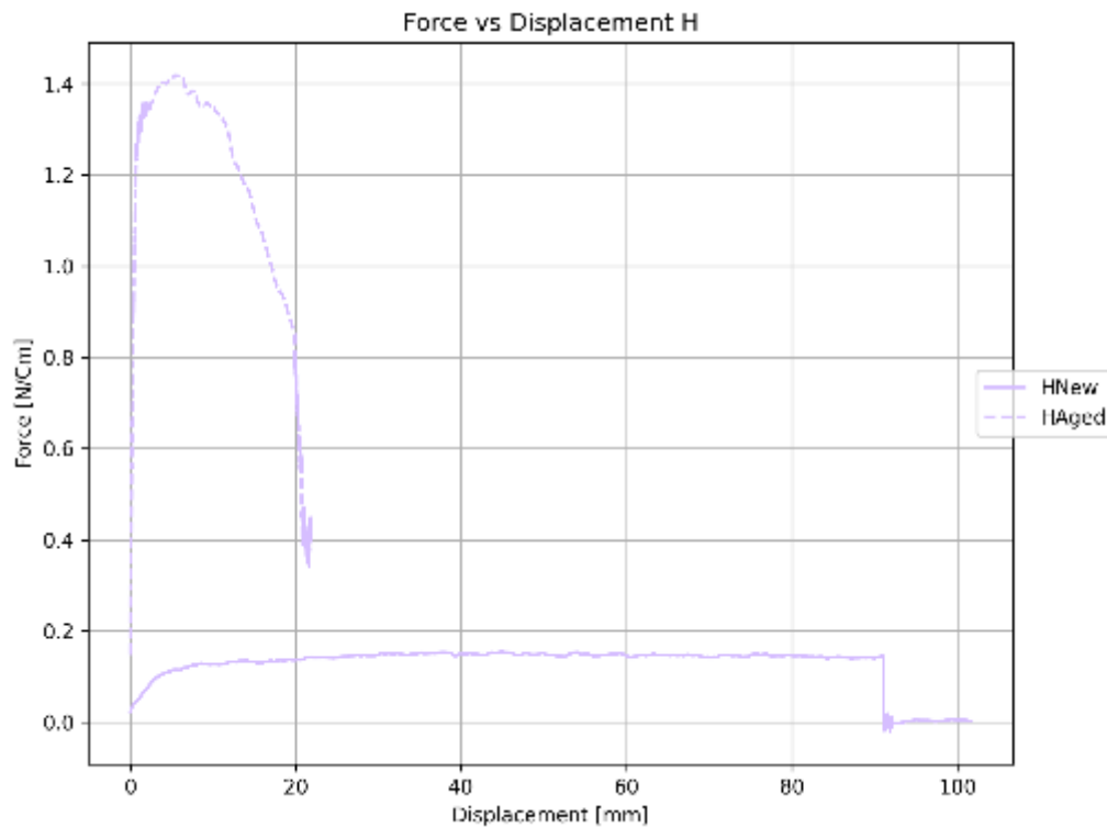
Figuur 5: krachtverplaatsingscurven van de afpeltests uitgevoerd op Coating H.
