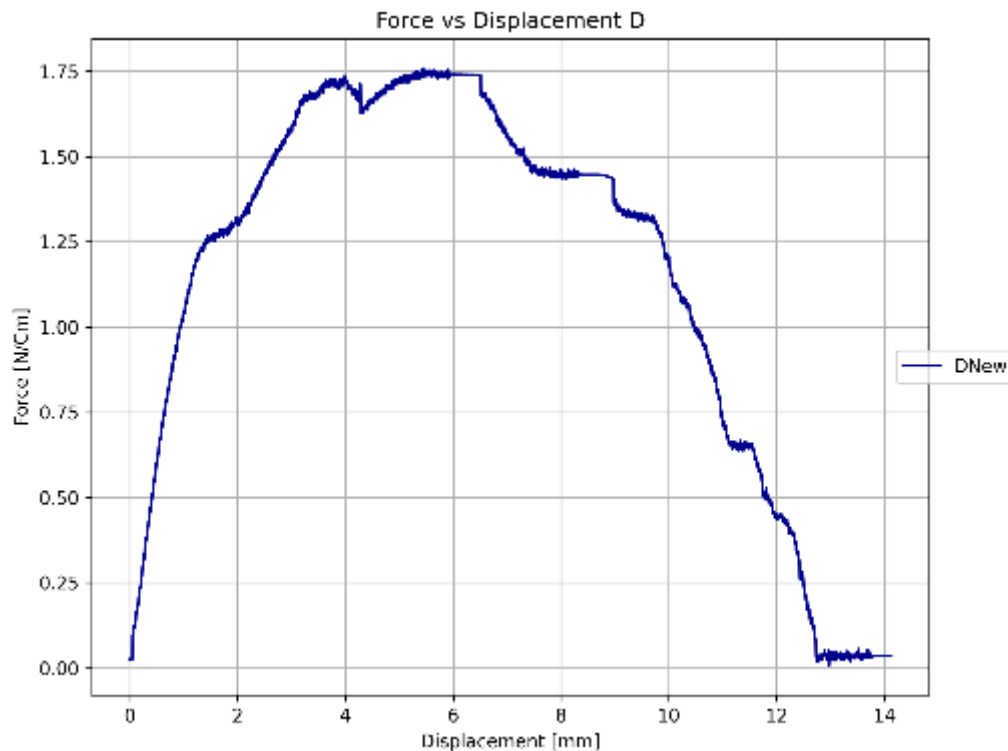
Figuur 4: krachtverplaatsingscurve van de afpeltest uitgevoerd op Coating D.
