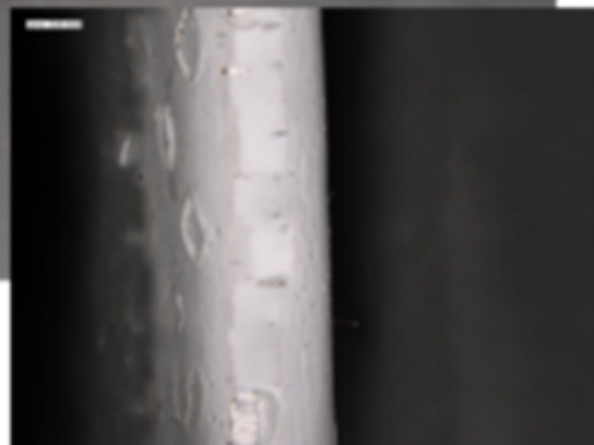
Figuur 7 microscopische beelden van de niet-verouderde en verouderde monsters van Coating D laten zien dat de coating scheurt bij T0.
